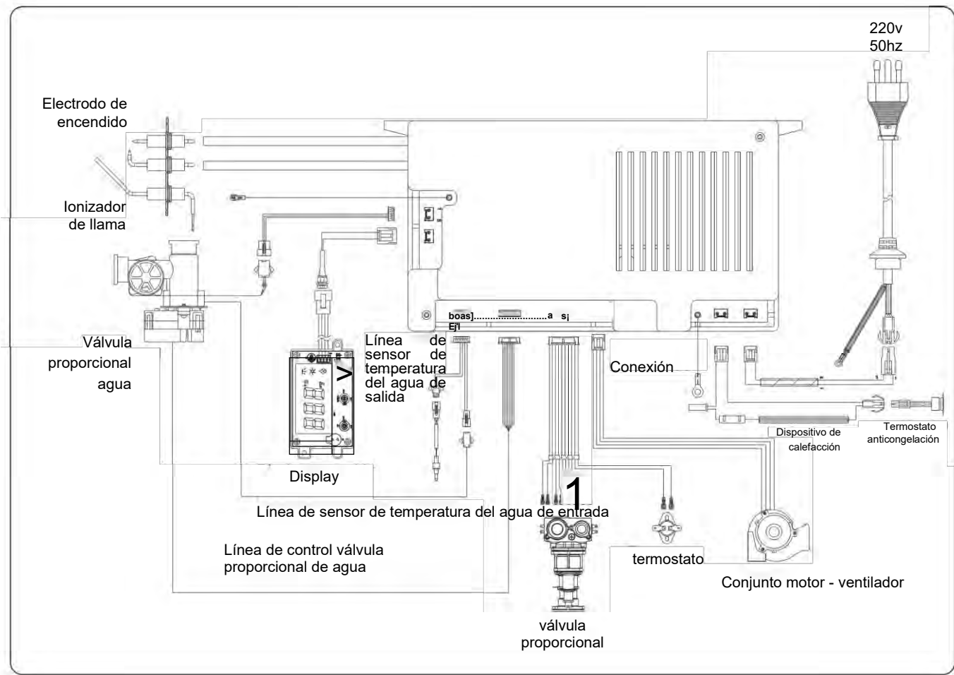
Diagrama Eléctrico
