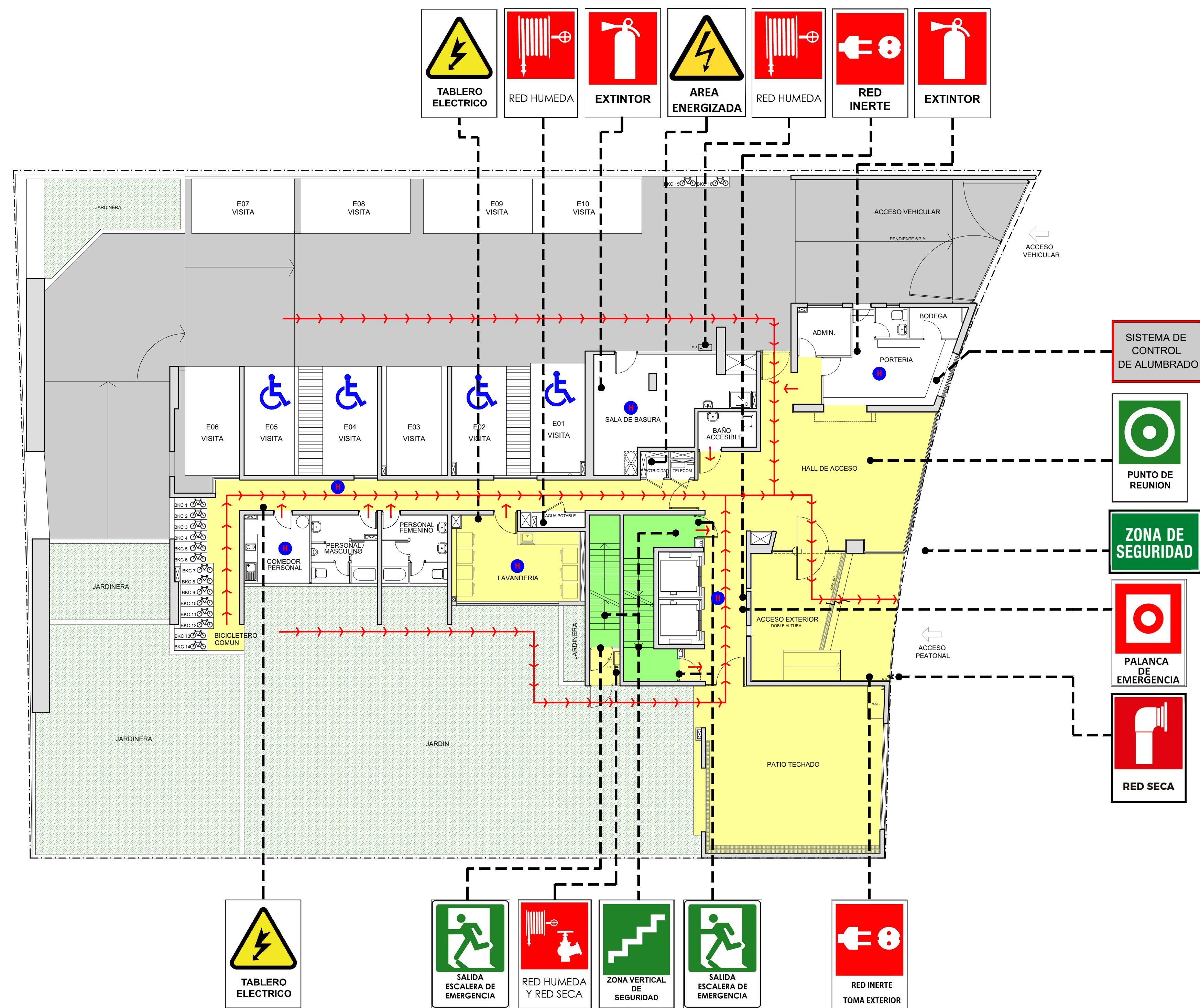
PLANTA PISO 1
