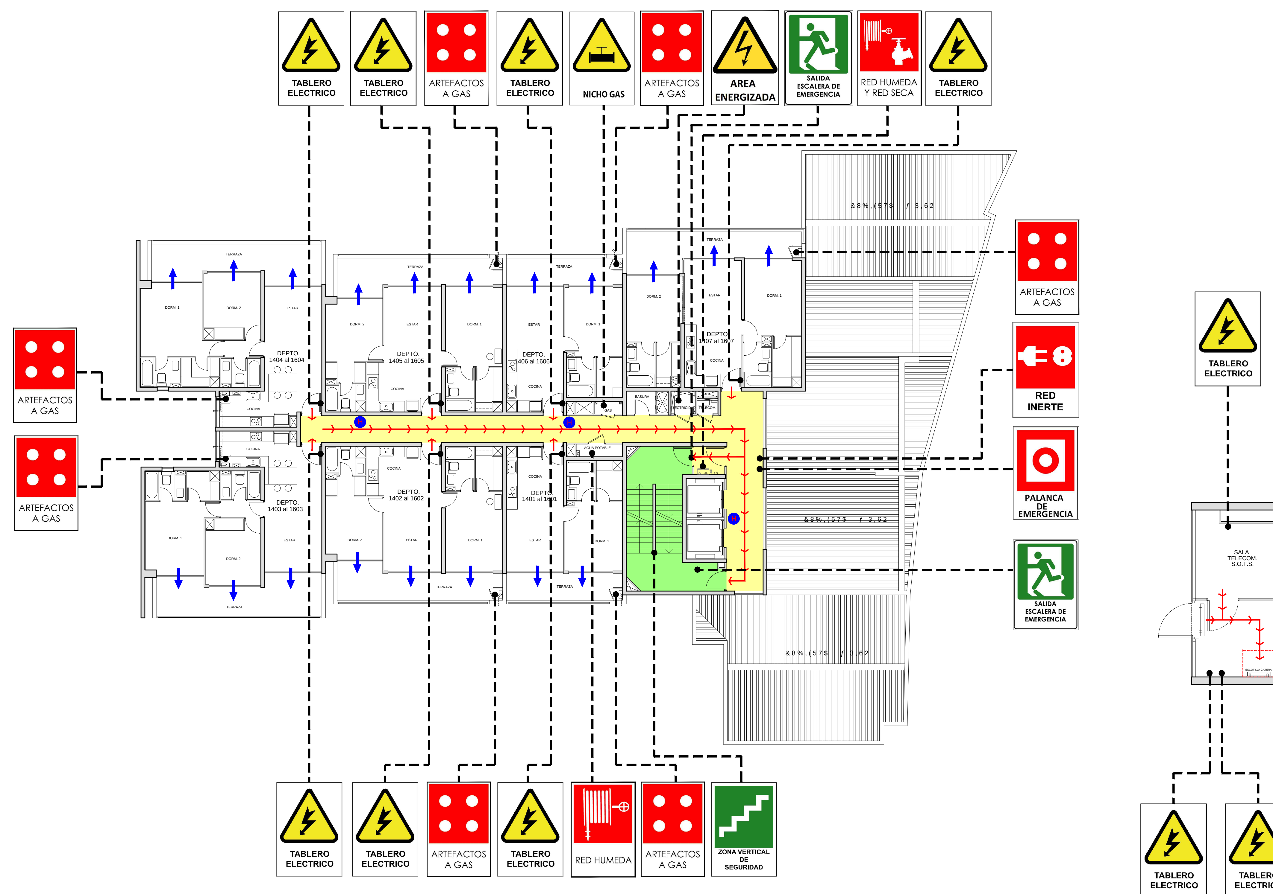
PLANTA PISOS 14 - 16
