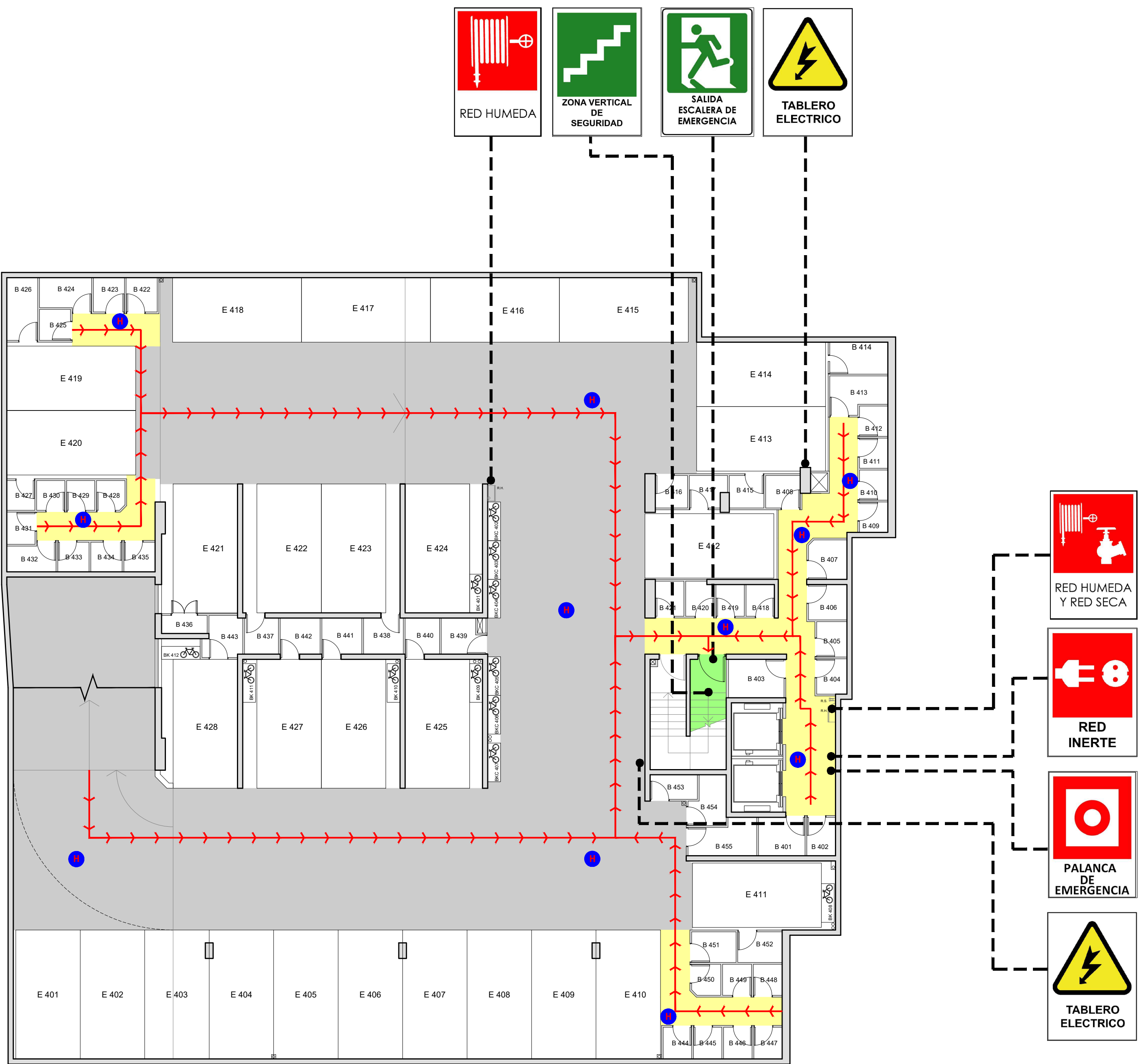
PLANTA SUBTERRANEO -4
