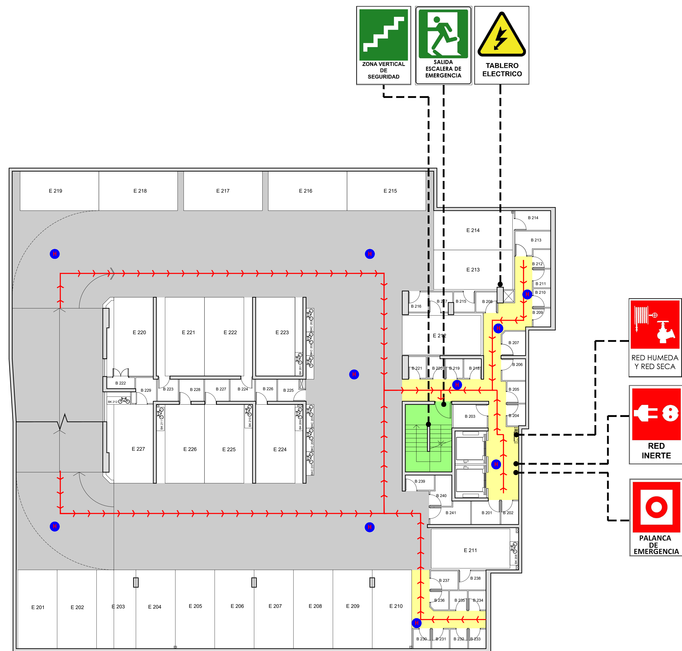
PLANTA SUBTERRANEO -2
