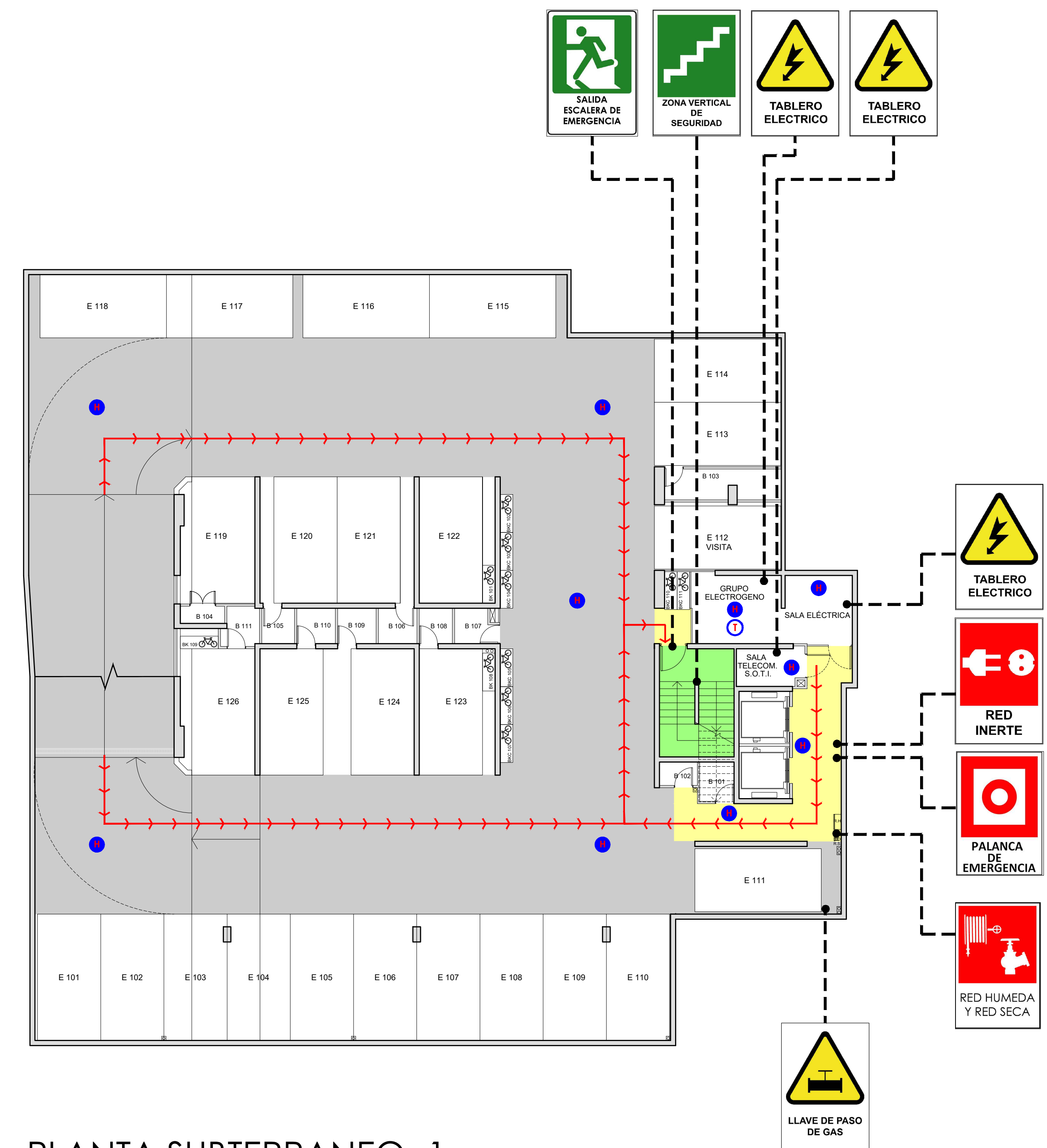
PLANTA SUBTERRANEO -1
