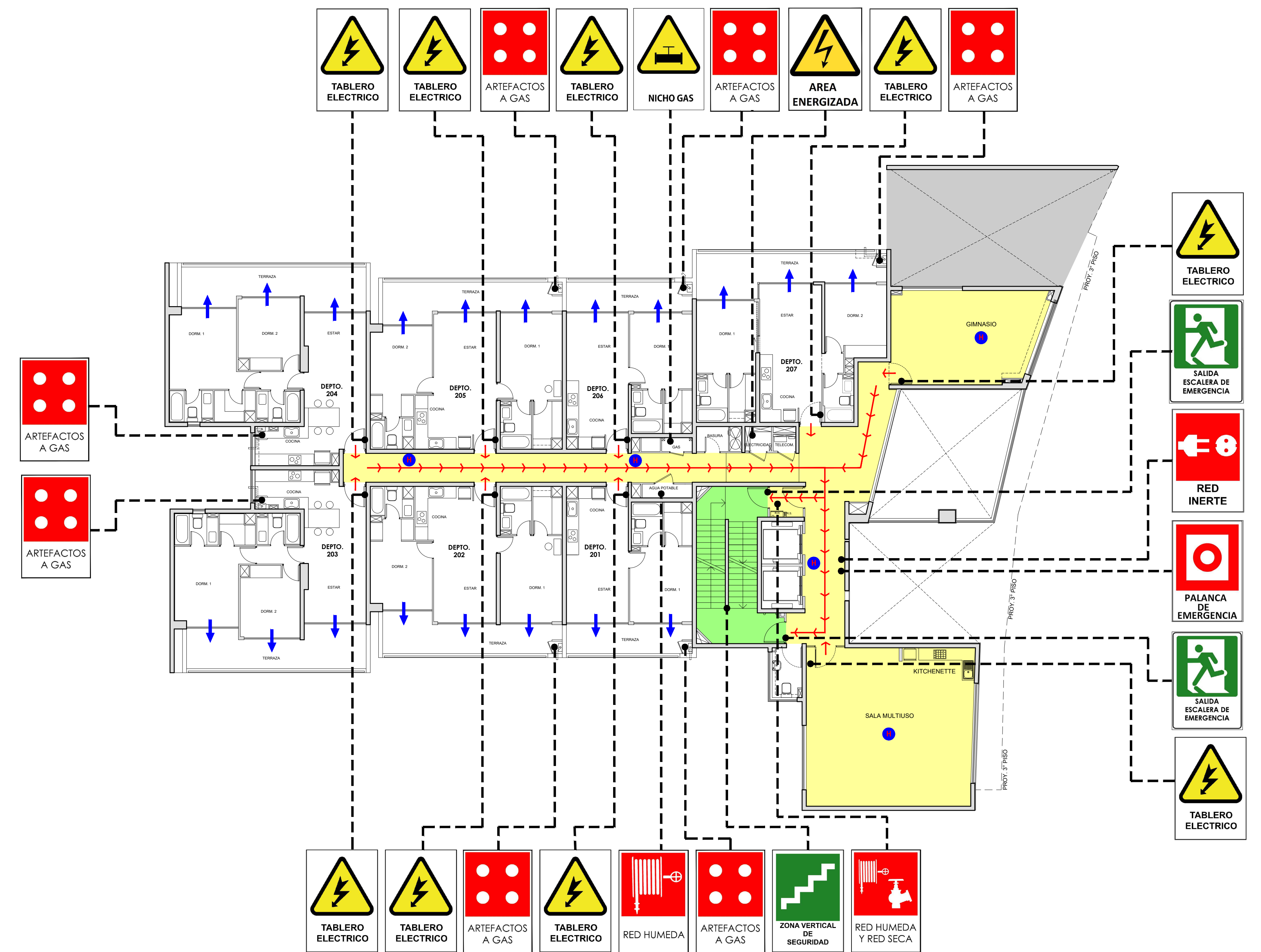
PLANTA PISO 2
