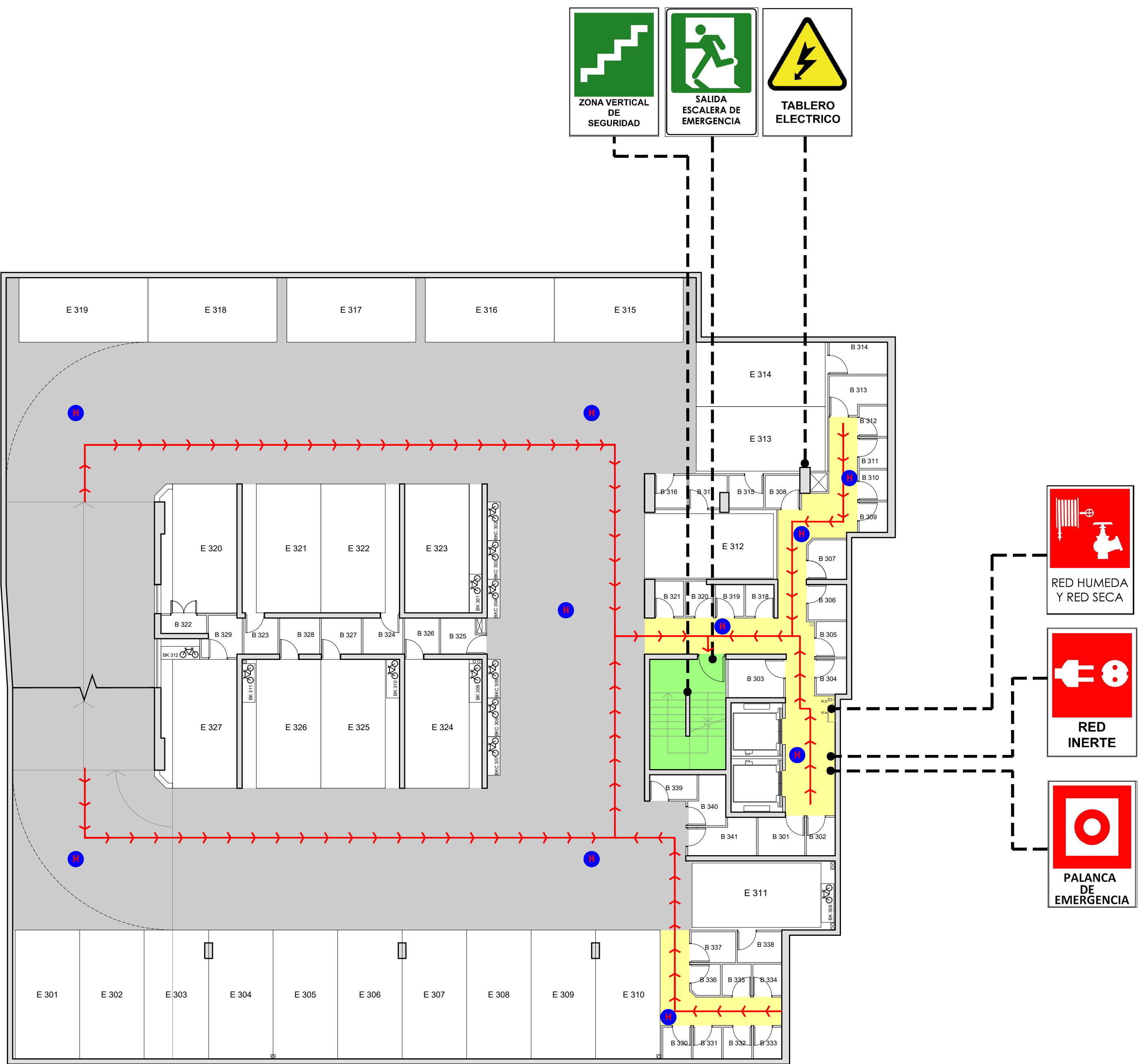
PLANTA SUBTERRANEO -3
