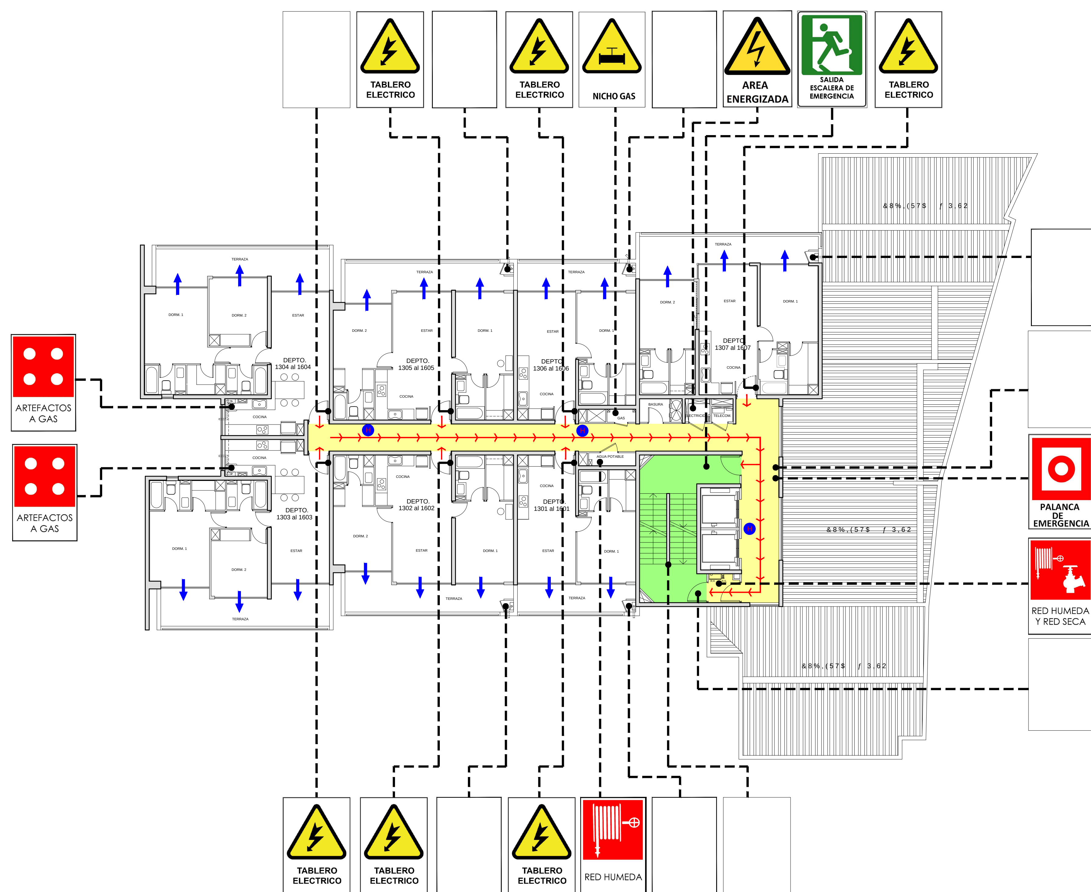
PLANTA PISOS 13 - 15
